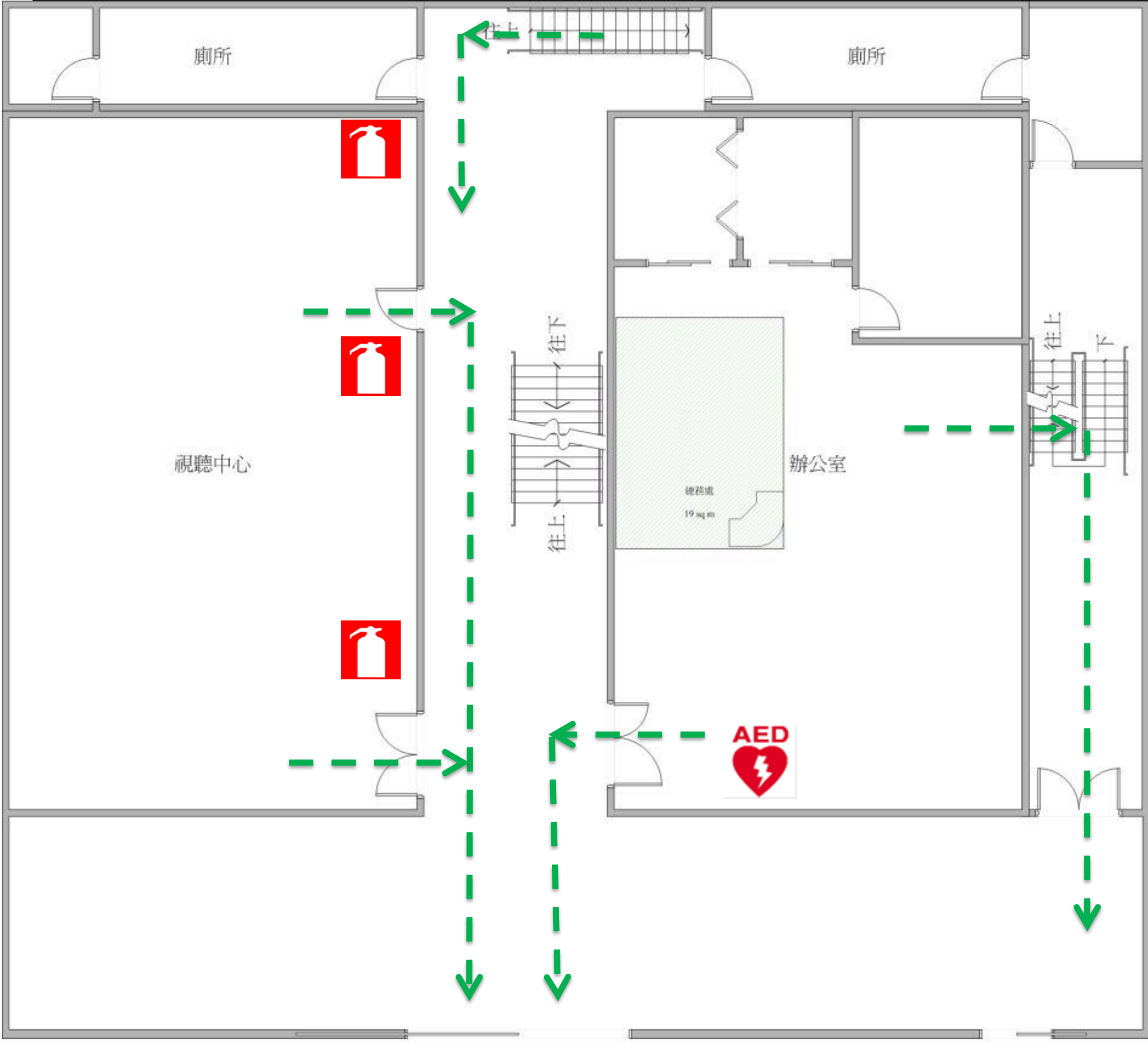
志仁高中行政大樓 1 樓平面圖 行政教學大樓1樓平面圖
