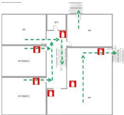
志仁高中行政大樓4樓平面圖 行政教學大樓4樓平面圖
