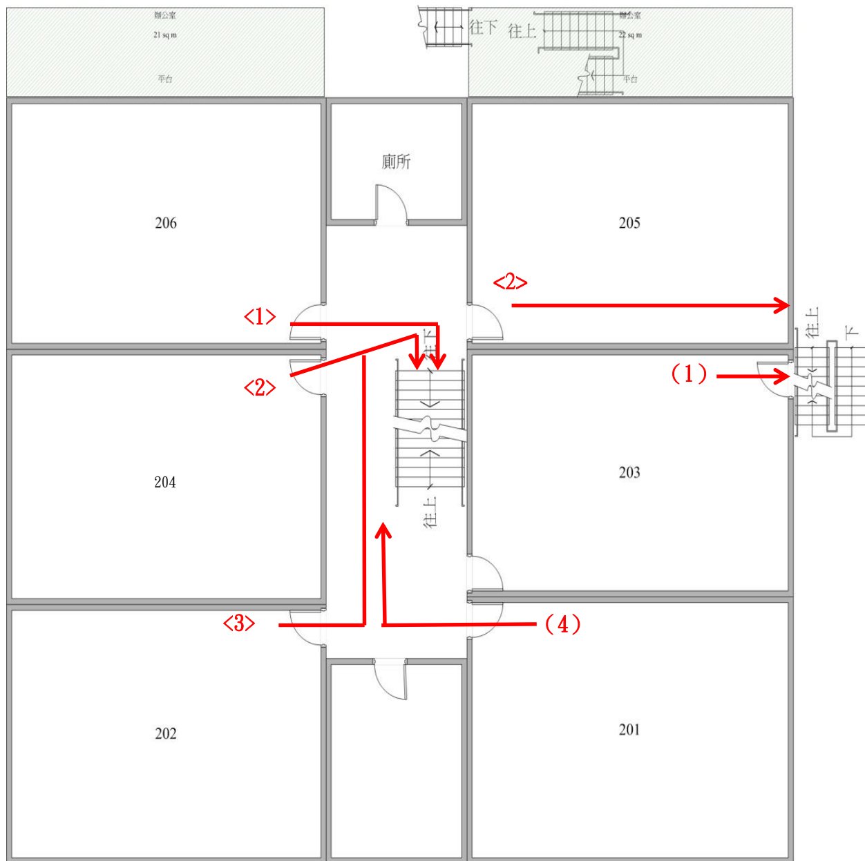
志仁高中行政大樓 2 樓平面圖
