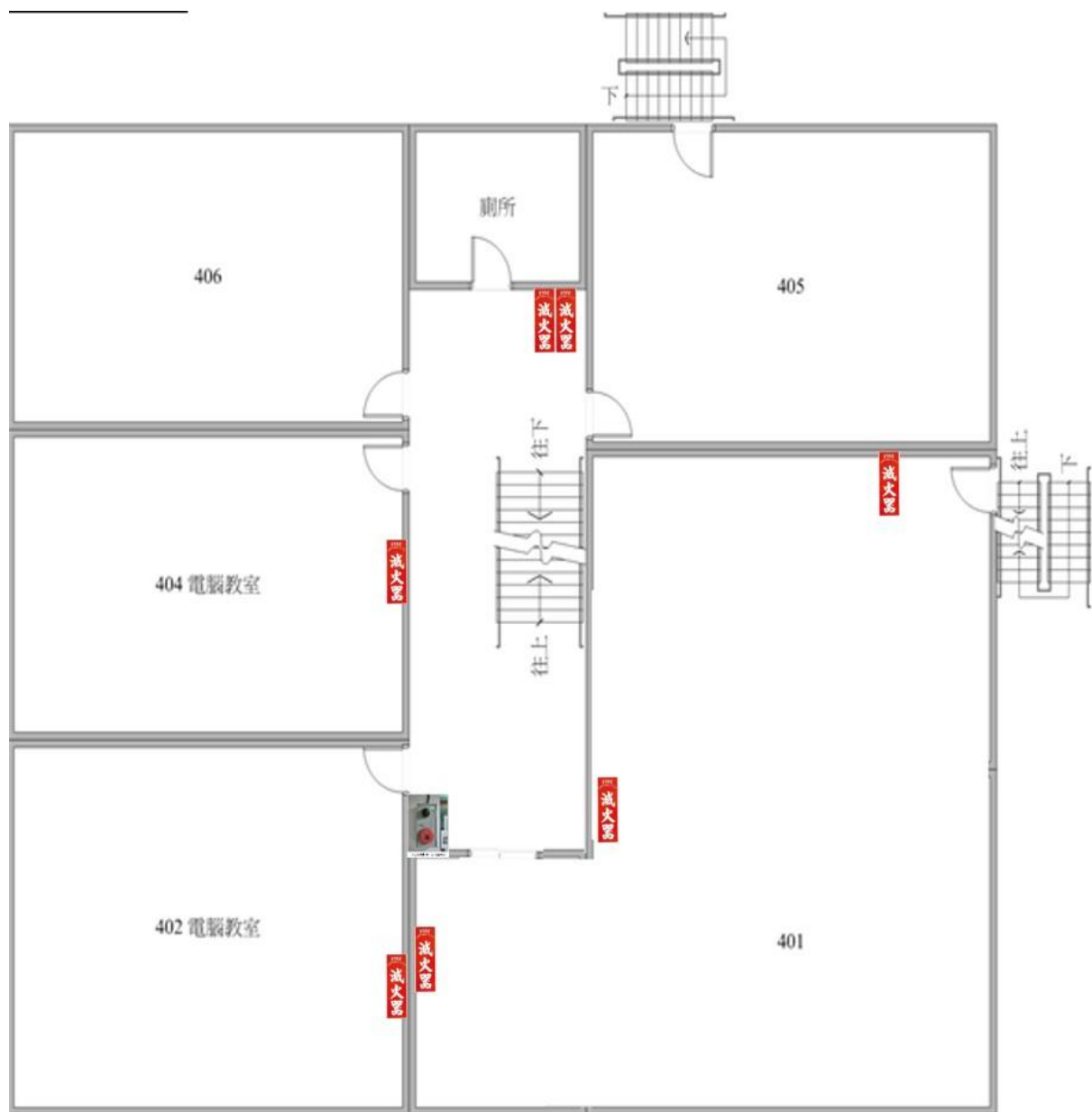
志仁高中行政大樓4樓平面圖暨滅火器分布圖
